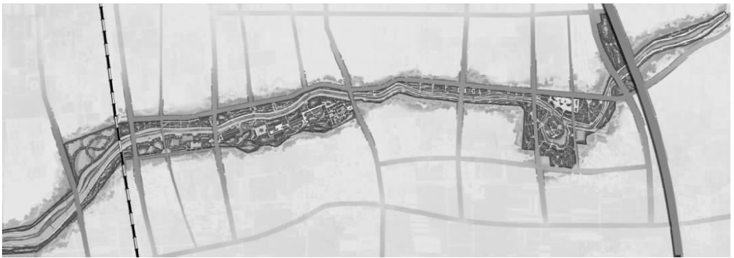
图1 华阴长涧河景观设计总平面图
